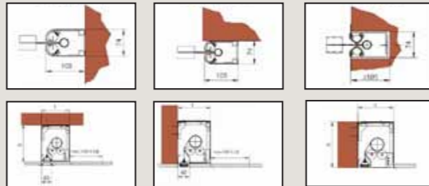
Ray ve sarım kutusu bağlantı tipleri
